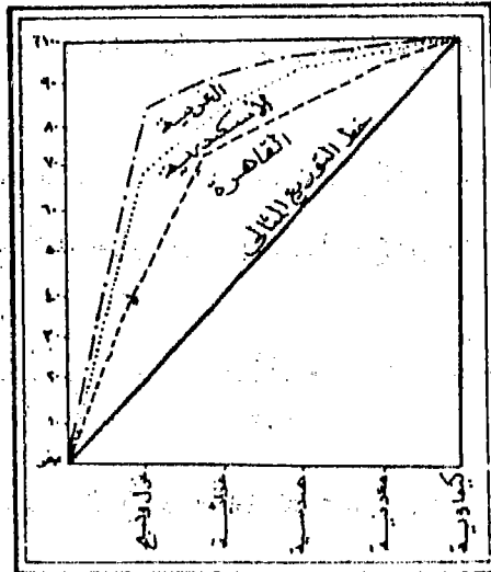
منحنى لورنز لقياس تنوع الصناعات في ثلاث مناطق جغرافية
